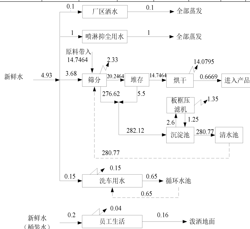
图 2-1 本项目水平衡图 \text{m}^3/\text{d}
