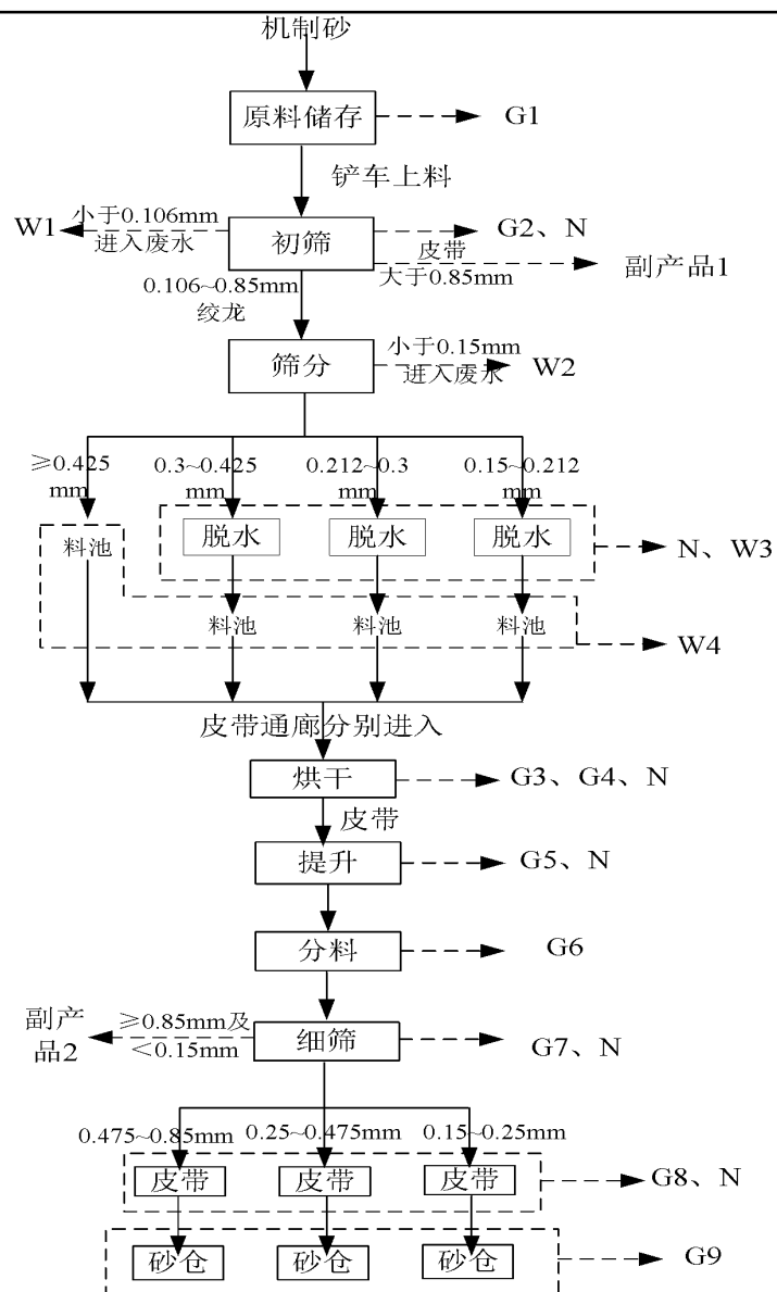
图 2-2 项目烘干砂生产工艺及排污节点图
