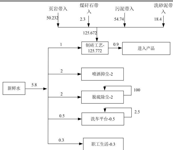
图 2-1 水量平衡图 (m³/d)
