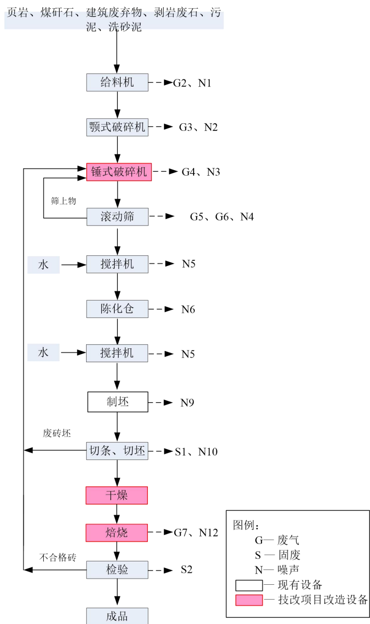
图 2-2 生产工艺流程及排污节点图
