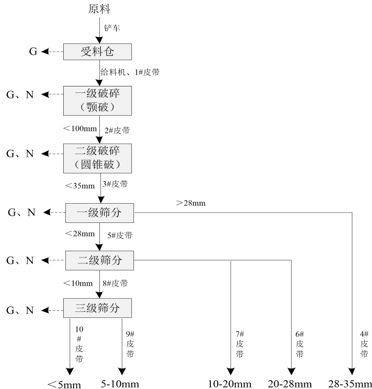
图 2-2 现有工程二期石渣生产线生产工艺流程及产排污节点图
