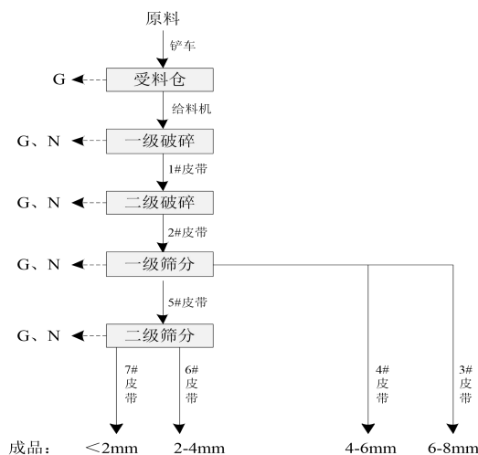
图 2-1 现有工程一期石渣生产线生产工艺流程及产排污节点图
