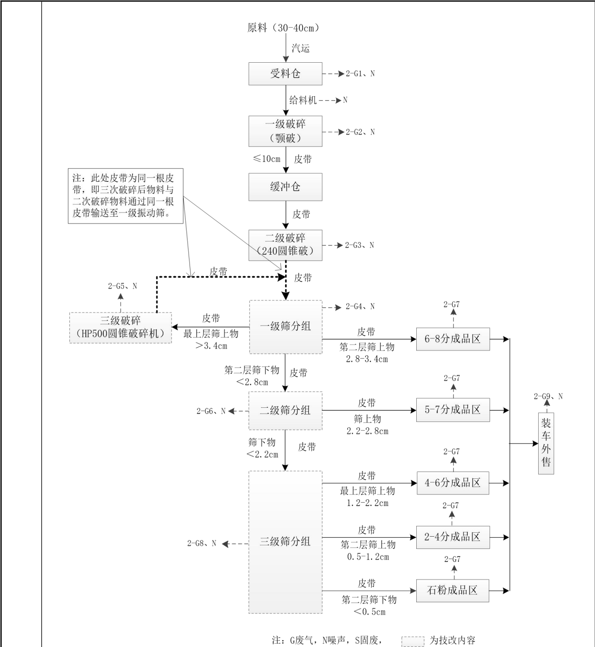
图 2-5 技改后二期石渣生产线工艺流程及产排污节点图
