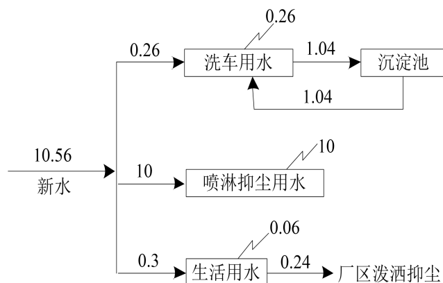
图 2-3 现有工程（一期+二期）给排水平衡图 单位：m³/d
