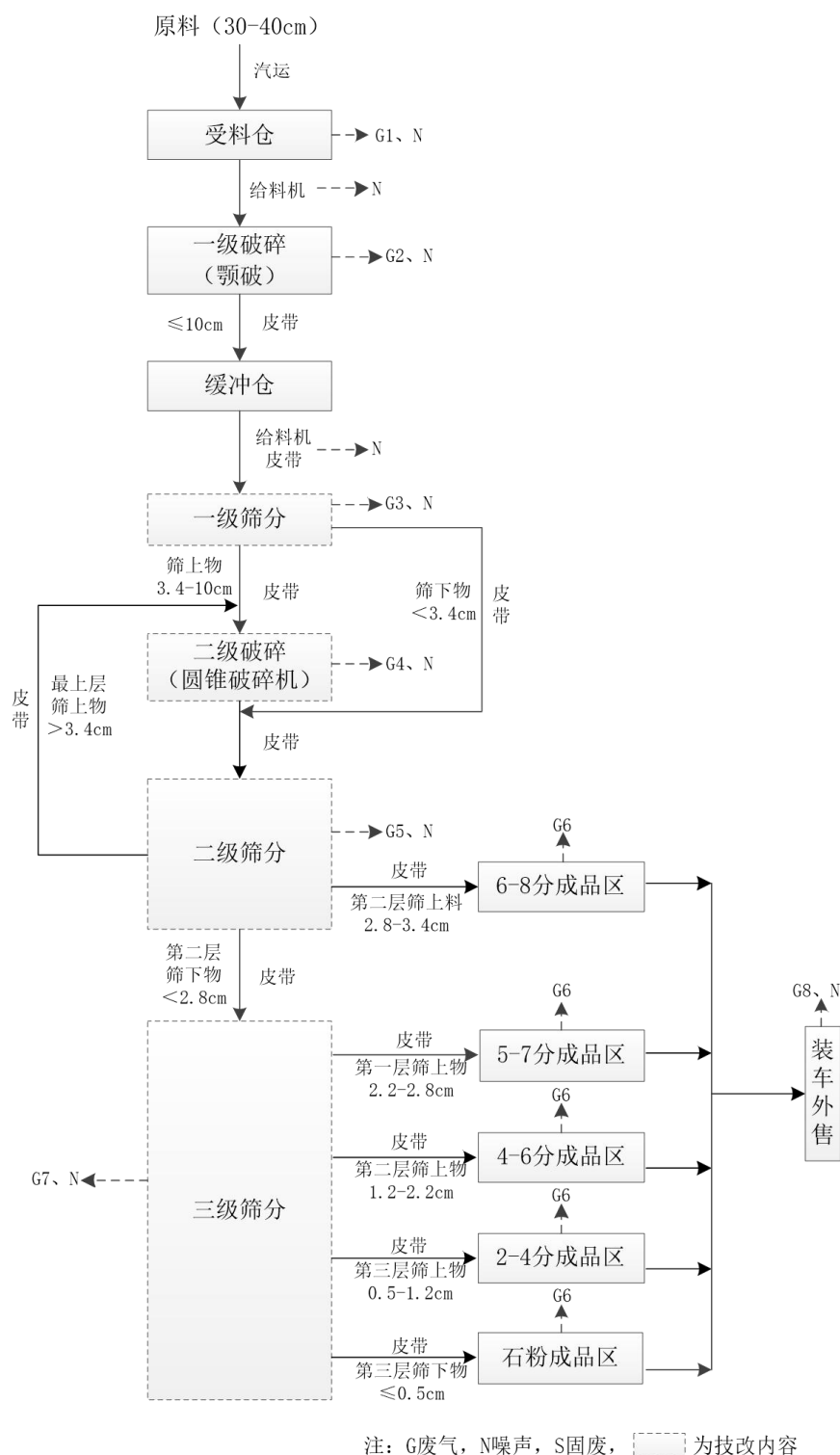
图 2-4 技改后一期石渣生产线生产工艺流程及产排污节点图
