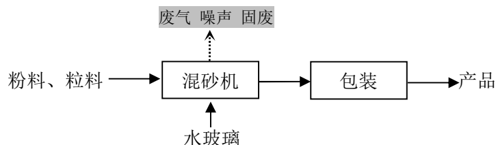
图 2-5 铁沟料混料生产工艺流程及产污节点图
