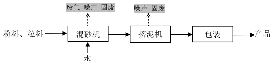
图 2-4 炮泥混料挤泥生产工艺流程及产污节点图
