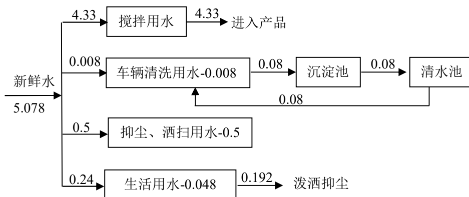
图 2-1 水平衡图 单位：m³/d
