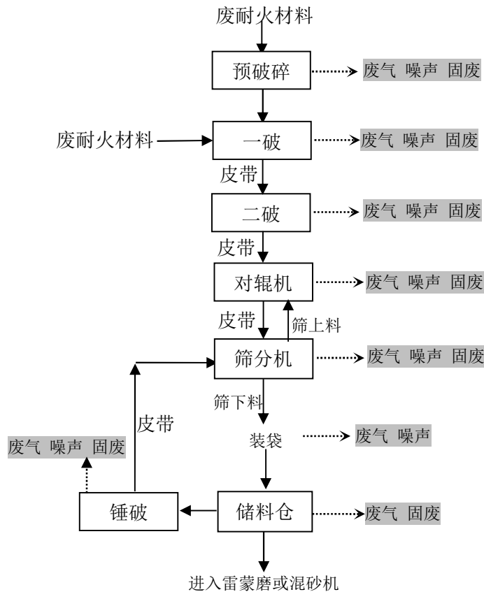
图 2-2 破碎筛分生产工艺流程及产污节点图
